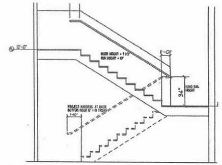
STAIR SECTION SCALE: 1/8"=1'-0"
